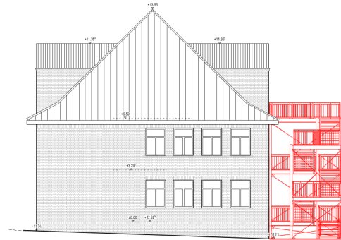
Ansicht Westen
