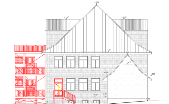
Ansicht Osten
