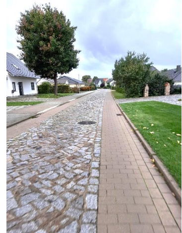
Abbildung 14: Beispiel für Radfahrbereiche auf Fahrbahnen mit Naturpflaster
