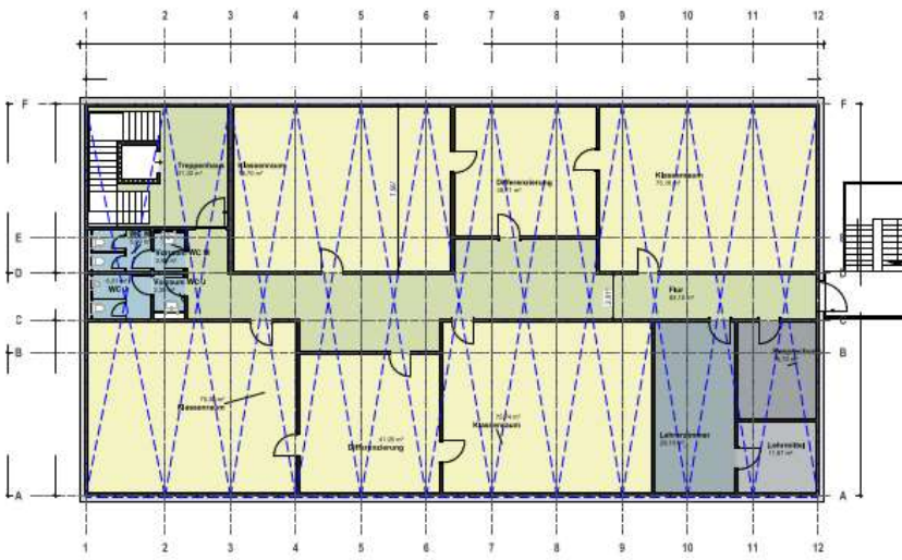
Grundriss Obergeschoss
