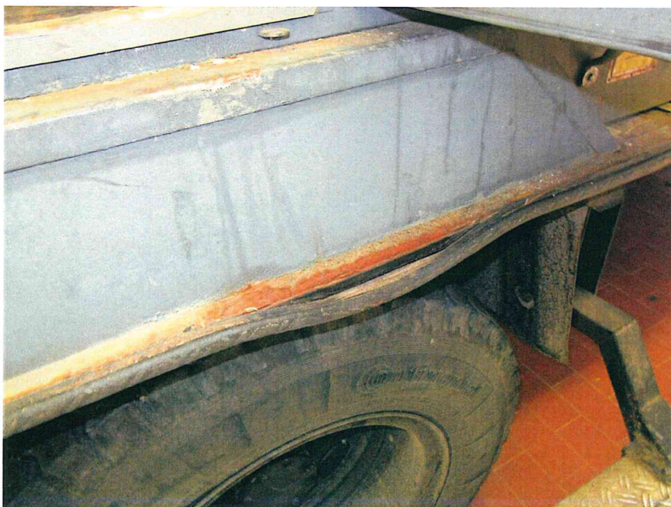
Bild 16 : Korrosion
