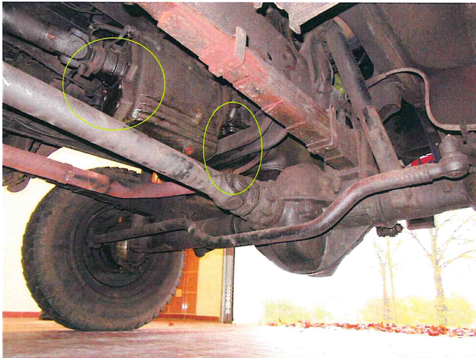
Bild 13 : Ölverlust leicht
