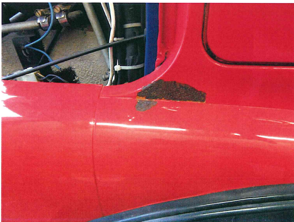
Bild 18 : Lackschaden/Korrosion
